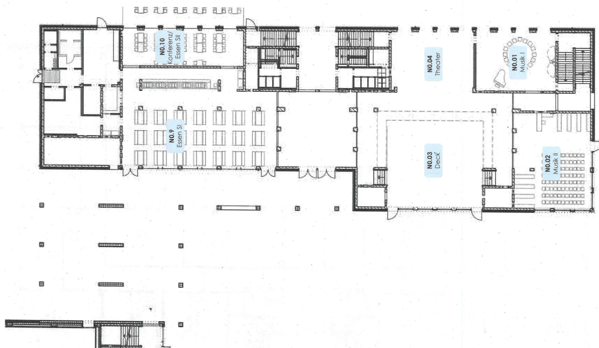
Raumplan Gymnasium Hoheluft – Neubau, Erdgeschoss
